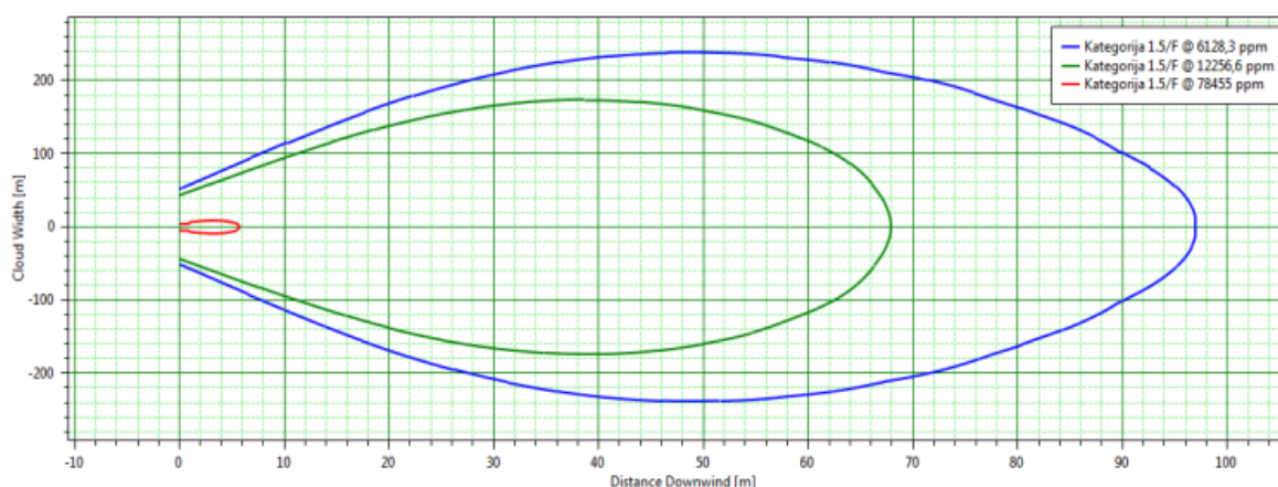
Slika 24. Obris oblaka para benzina sa zonama GGE, DGE, 50DGE
