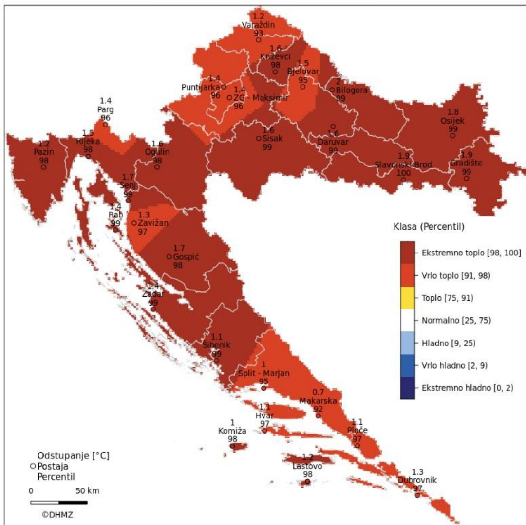
Godina 2023. Srednja temperatura zraka Percentili u odnosu na normalu 1991.-2020.
